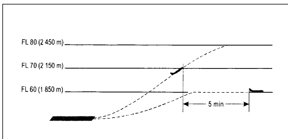
Rysunek 5-39. Separacja pięcioczynowa między odlatującymi statkami powietrznymi lecącymi po tej samej linii drogi (patrz pkt 5.6.3.)
