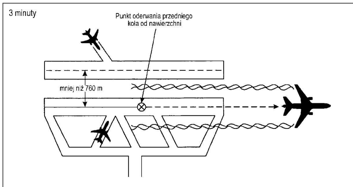
Rysunek 5-43. Separacja trzyminutowa między statkami powietrznymi lecącymi po tej samej linii drogi i która jest uwarunkowana turbulencją w śladzie aerodynamicznym (patrz pkt 5.8.3.2.)
