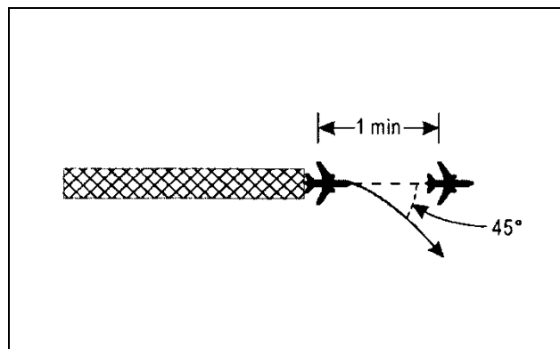
Rysunek 5-37. Separacja jednoczynowa między odlatującymi statkami powietrznymi z kątami drogi różniącymi się nie mniej niż 45° (patrz pkt 5.6.1.)
