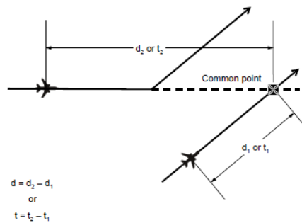
Rysunek 5-32. Obliczanie odległości podłużnej / czasu między statkami powietrznymi – ta sama zamierzona droga, ale nie jednakowa (patrz 5.4.2.9.5 b))
