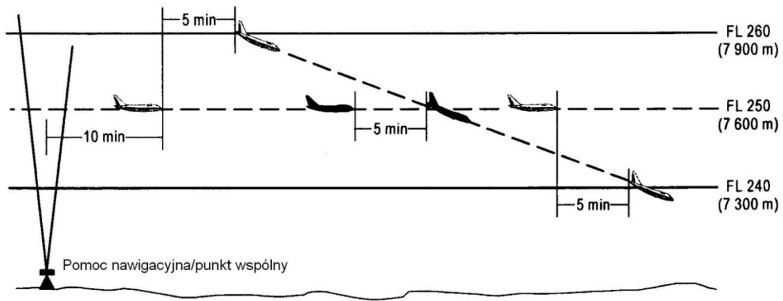
Rysunek 5-18B. Separacja pięciominutowa między statkami powietrznymi podczas zniżania i na tej samej linii drogi (patrz pkt 5.4.2.2.2.1. lit. c))
