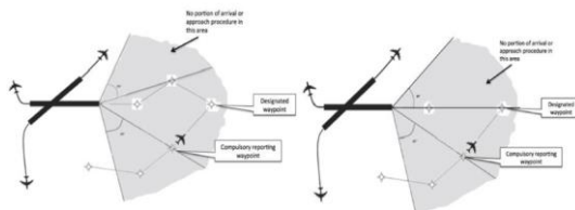
Rysunek 5-41 Przykłady obszaru ochrony przylotowej
