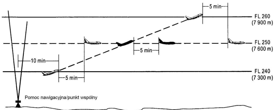
Rysunek 5-18A. Separacja pięciminutowa między statkami powietrznymi podczas wznoszenia i na tej samej linii drogi (patrz pkt 5.4.2.2.2.1. lit. c))
