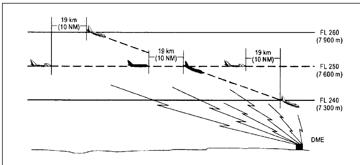
Rysunek 5-25B. Separacja — przy wykorzystaniu DME lub GNSS — 19 km (10 NM) między statkami powietrznymi podczas zniżania na tej samej linii drogi (patrz pkt 5.4.2.3.2.3. lit. c))
