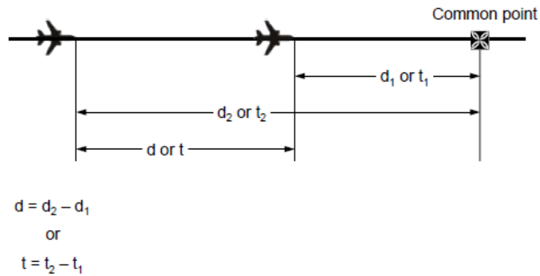
Rysunek 5-29. Obliczanie odległości podłużnej / czasu między statkami powietrznymi – jednakowa droga, ten sam kierunek (patrz 5.4.2.9.5 a))
