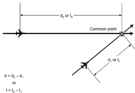
Rysunek 5-31. Obliczanie odległości podłużnej / czasu między statkami powietrznymi – ta sama droga, ale nie jednakowe i przecinające się drogi (patrz 5.4.2.9.5 b))
