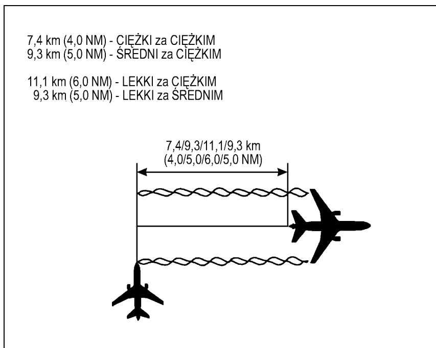
Rysunek 8- 1B. Statek powietrzny przecina ślad turbulencyjny drugiego statku powietrzego (patrz pkt 8.7.3.4. i 8.7.3.4.1.)
