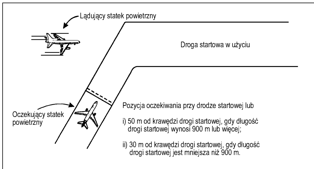
Rysunek 7- 2. Sposób oczekiwania statku powietrznego
