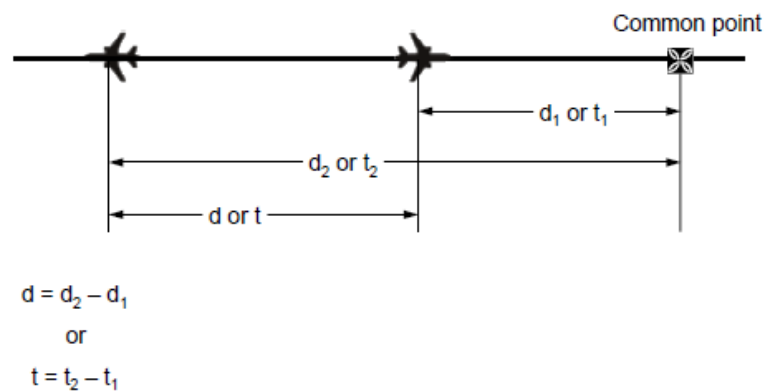
Rysunek 5-30. Obliczanie odległości podłużnej / czasu między statkami powietrznymi – jednakowa droga, przeciwny kierunek (patrz 5.4.2.9.5 a))
