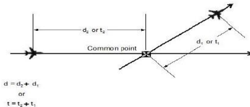
Rysunek 5-33. Obliczanie odległości podłużnej / czasu między statkami powietrznymi – przeciwne strony wspólnego punktu (patrz 5.4.2.9.5 b))
