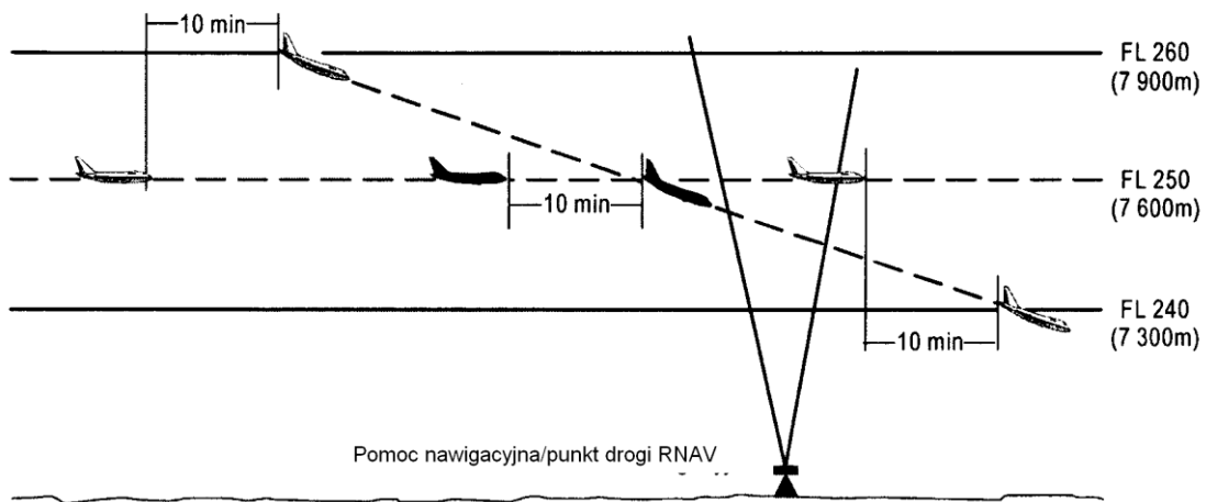
Rysunek 5-17B. Separacja dziesięciminutowa między statkami powietrznymi podczas zniżania i na tej samej linii drogi (patrz pkt 5.4.2.2.2.1. lit. b))
