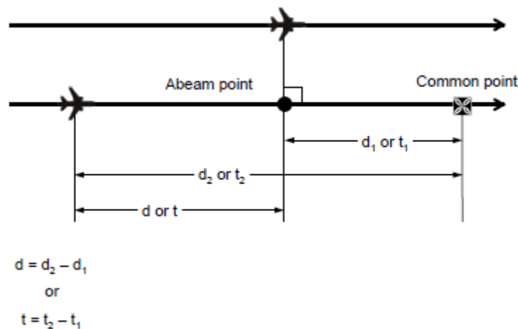
Rysunek 5-34. Obliczanie odległości podłużnej / czasu między statkami powietrznymi – równoległe drogi (patrz 5.4.2.9.5 c))
